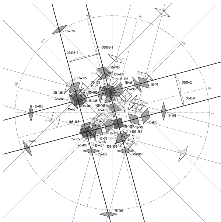
図 18 適当なオフセット距離に平行移動したゾーンストレートラインとゾーンストレートラインの交点に対応する菱形の配置
